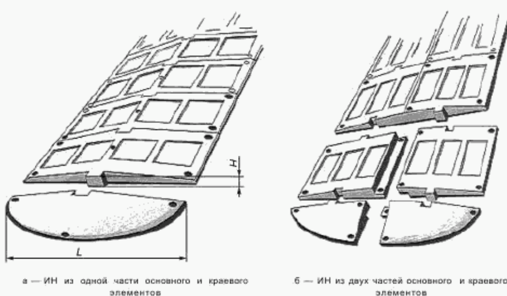
Рисунок 3 — Конструкция сборно-разборной ИН
